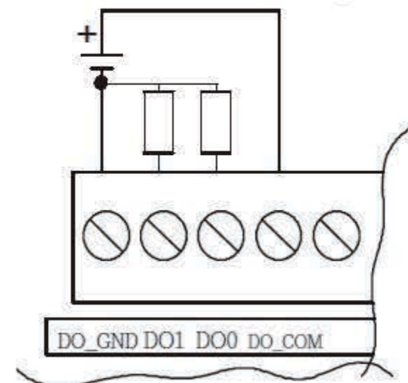
5190D/5190 Output
