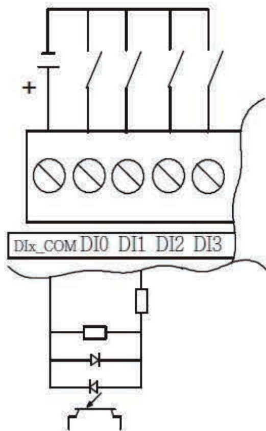
NPN Input
